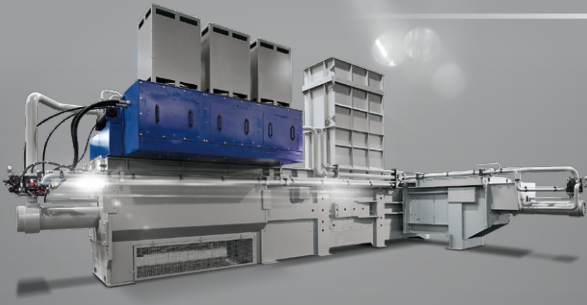
PRESSE Á COFFRE DE LA GAMME UPAMAX®
